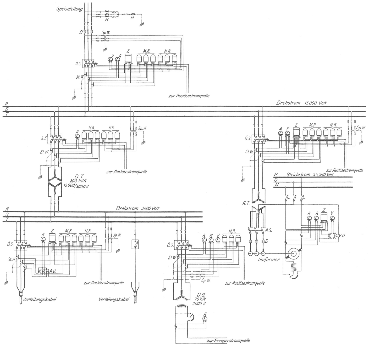
Abb. 165. Elektrizitätswerk Hartha mit Transformator für 15 000/3000 Volt.
