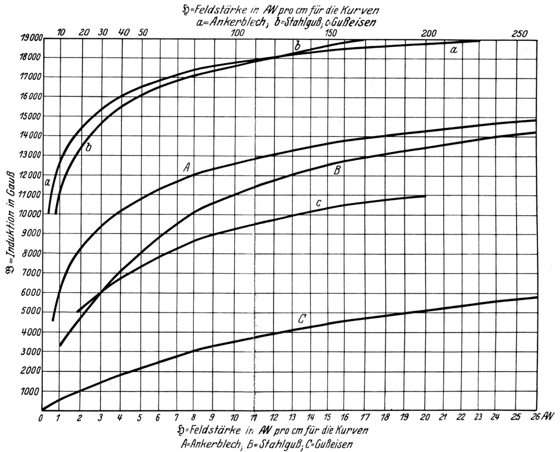
Magnetisierungskurven für Ankerblech, Stahlguß und Gußeisen.
