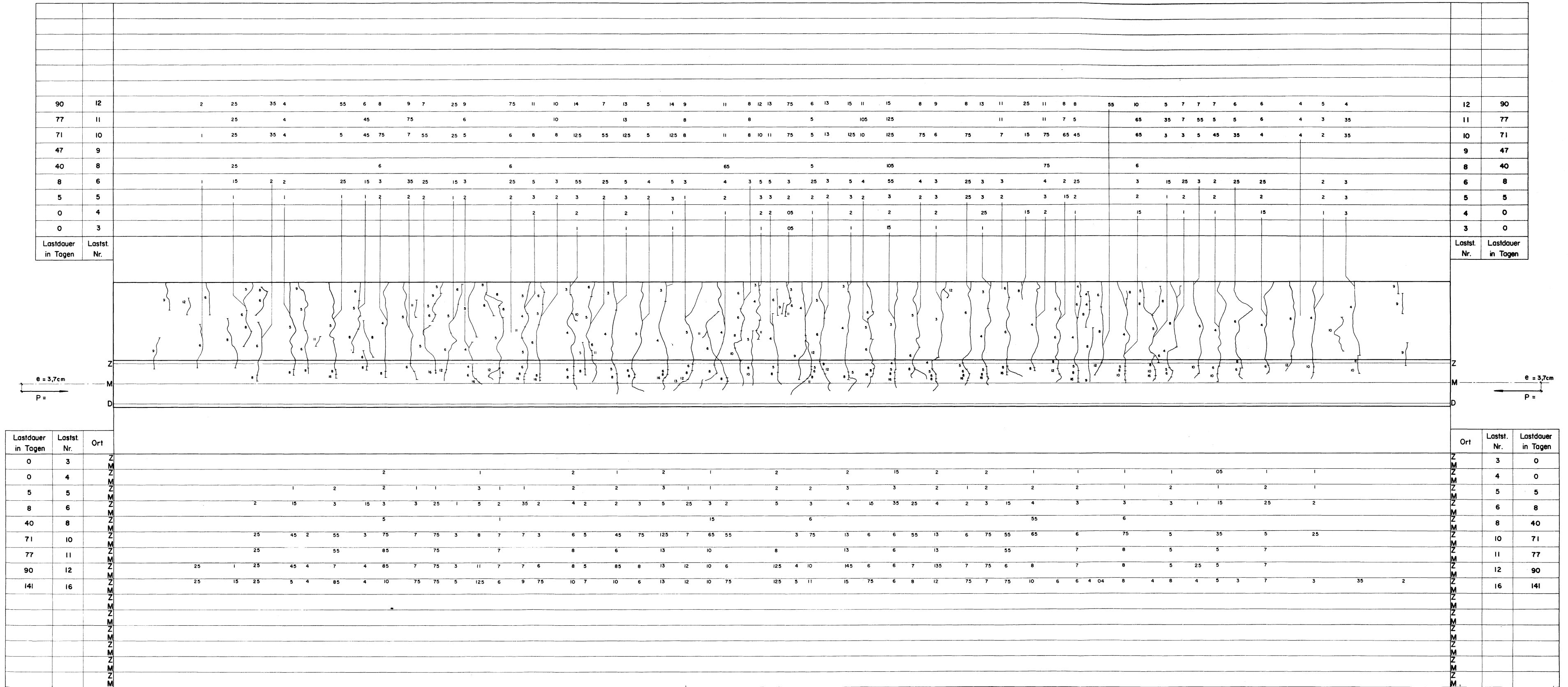
Bild 11 : Risseplan der Stütze 25 (M. 1:10 , Rissbreiten in 1/100 mm)
